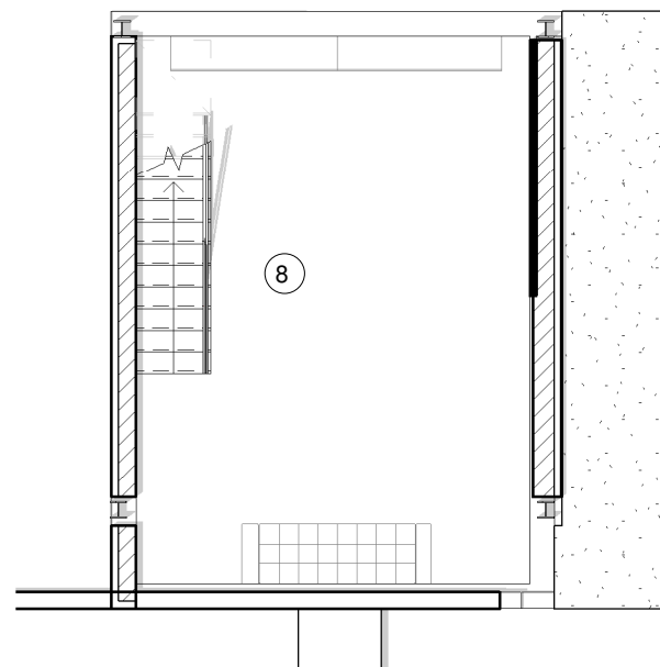
PLANTA SEMISÓTANO
