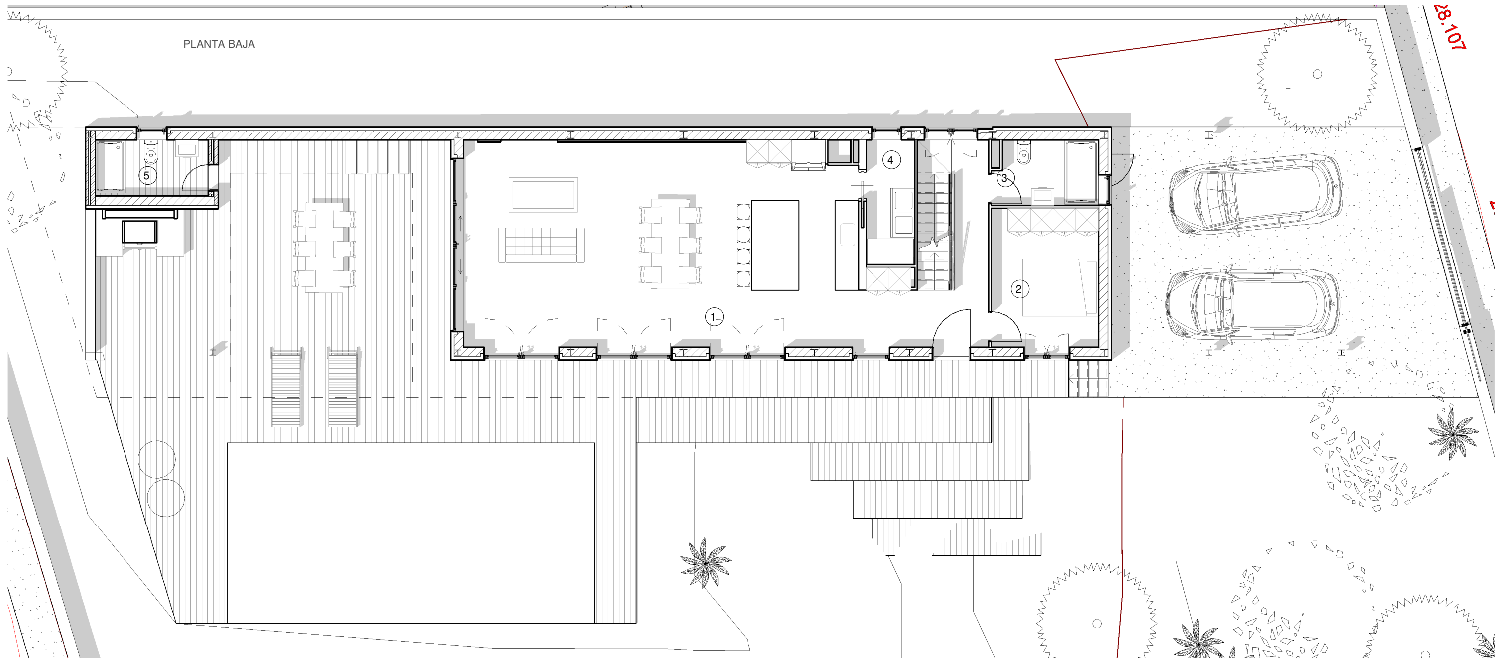
Planta baja y semisótano - superficie útil
